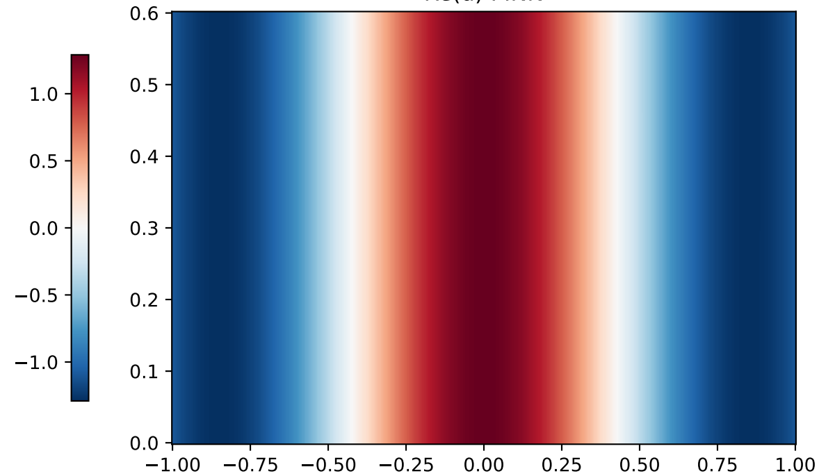
Re(u) PINN
